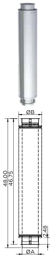
48" Fixed Length / DWFLØ-48L
