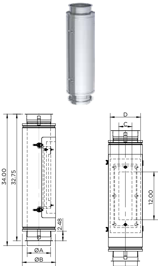
Inline Access Door Length / DWFLØ-IAD
