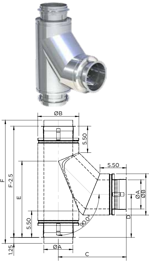
90° Grease Boot Tee / DWFLØ-87GBT
