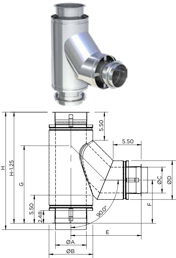
90° Reduction Boot Tee / DWFLØ-90BTØ
