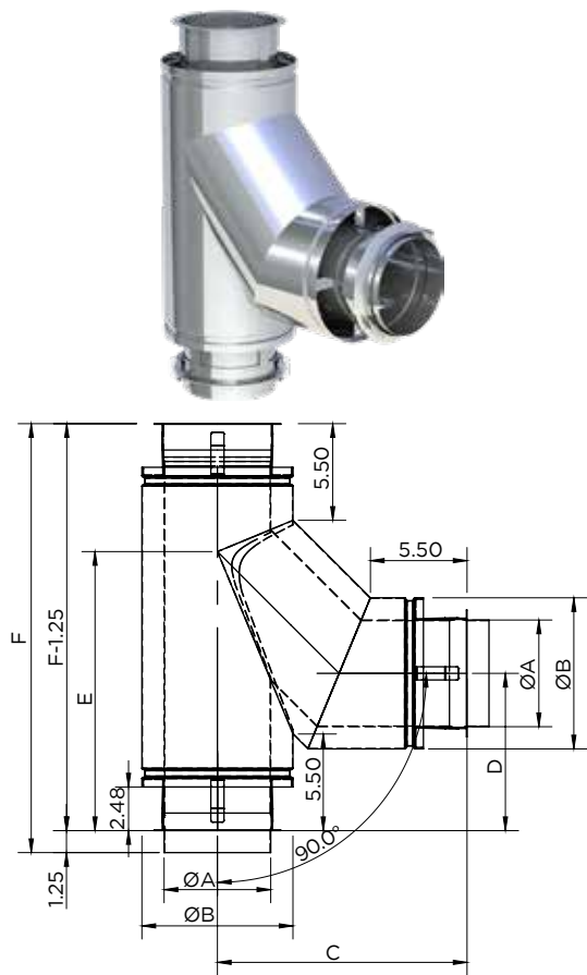
90° Boot Tee / DWFLØ-90BT
