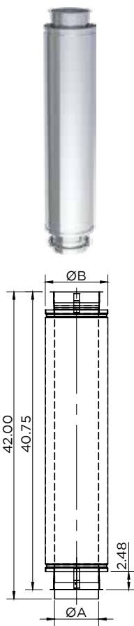
42" Fixed Length / DWFLØ-42L
