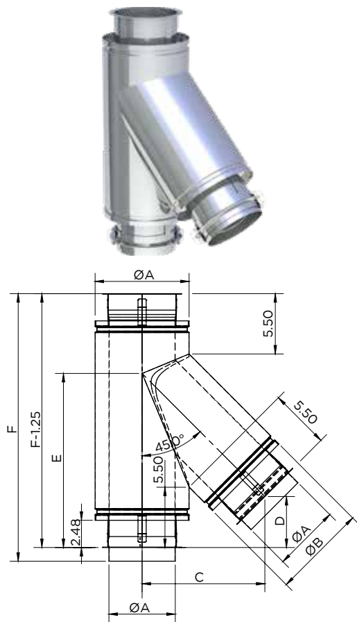
45° Tee / DWFLØ-45T
