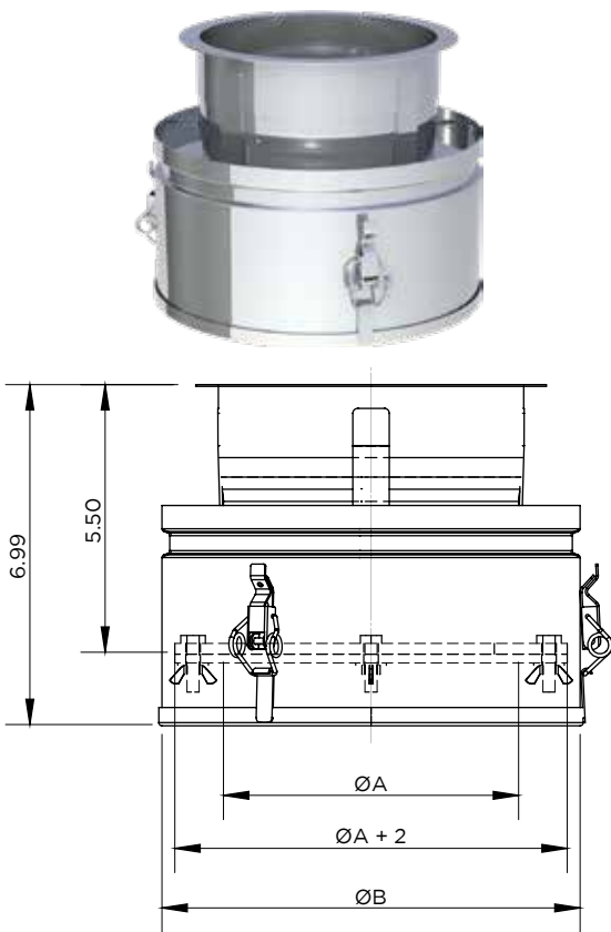
Grease Tee Cap Access / DWFLØ-GTCA
